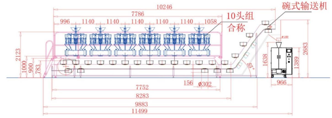
颗粒混合物料生产线 Pellet mixture production line
